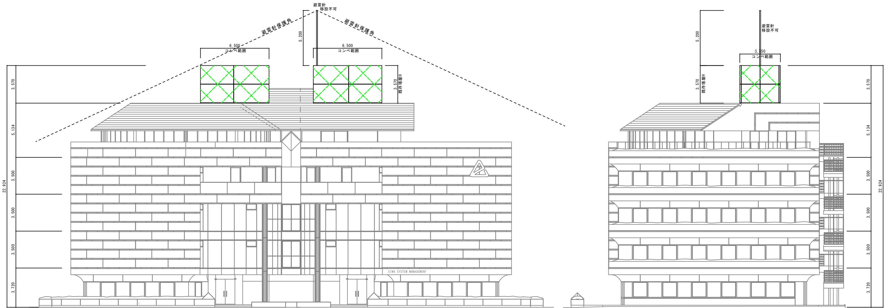
西面立面图 S 1/150
